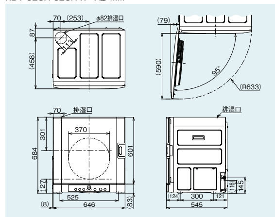
RDT-52SA・52SA-R 単位:mm
