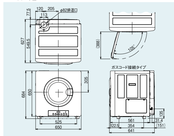
RDT-80 単位:mm
