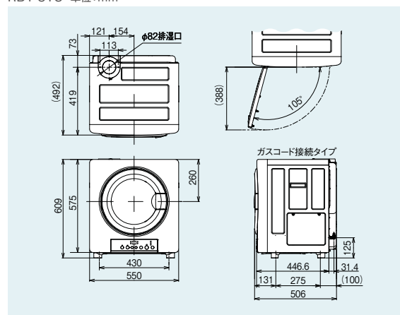
RDT-31S 単位:mm
