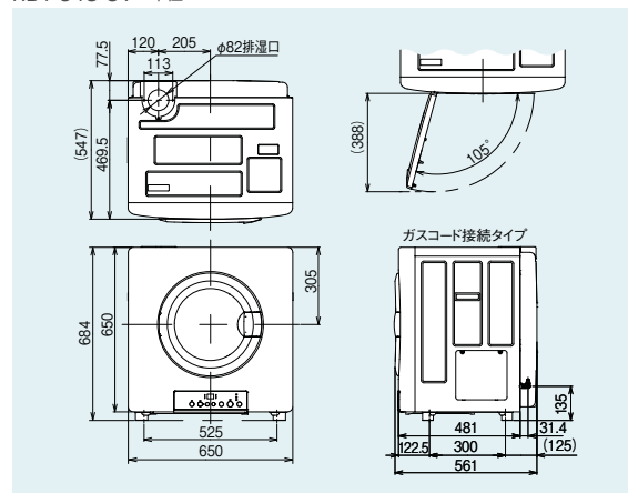
RDT-54S-SV 単位:mm
